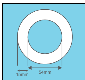
Protectube simples e blindado (15x54mm).
